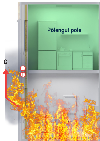
Paigaldatud Firebreather® Cavity Barrier
